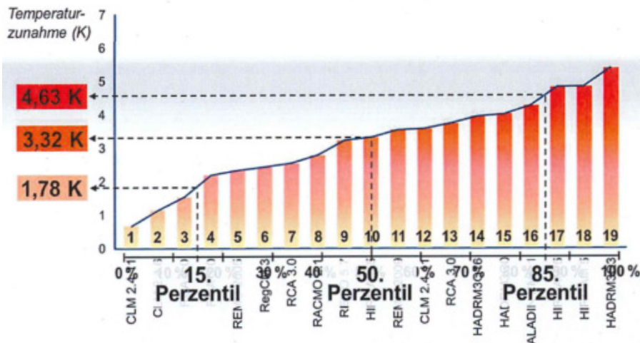
Abb. 6. Einteilung von Werten in Perzentile.
